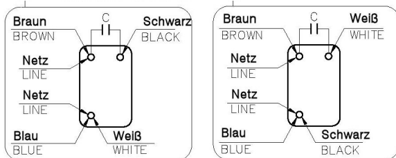
linksl. Pumpe auf Welle gesehen rechtsl. Pumpe auf Welle gesehen
