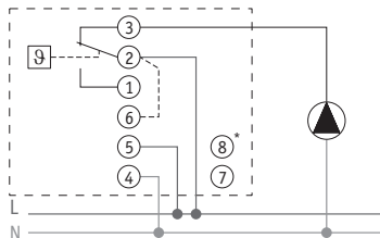
Commande d'un circulateur ou d'une vanne électrothermique
