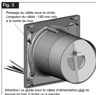
Attention: Le guide pour le câble d'alimentation doit se trouver en bas à droite ou à gauche
