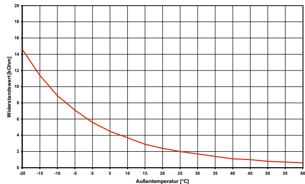
Abb. 9.2: Fühlerkennlinie NTC-2 nach DIN 44574 Außentemperaturfühler
