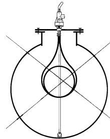
Bild 5: Falsche Montage
