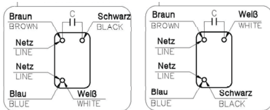
links. Pumpe auf Welle gesehen
