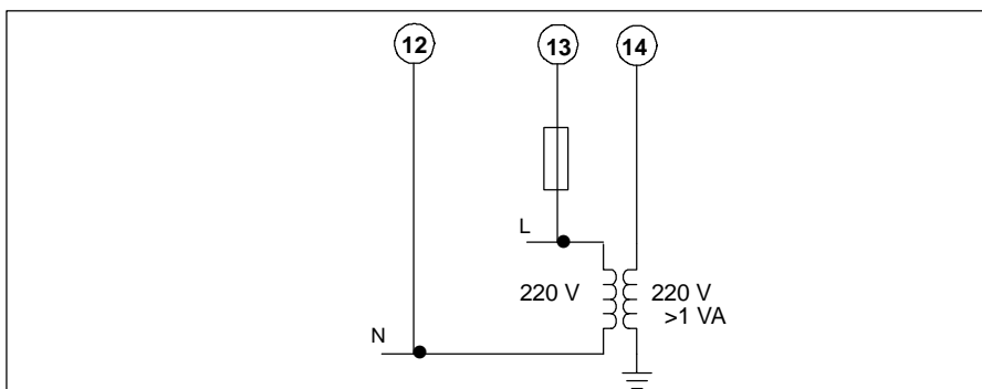
Fig. 3 Application of S4570AS/BS/LS to floating mains Verwendung von S4570AS/BS/LS in einer Schwebungsnetz Toepassing van S4570AS/BS/LS in een zwevend net
