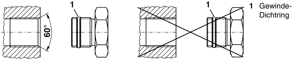
Bild 1: Richtig: Muttergewinde anfasen Bild 2: Falsch
