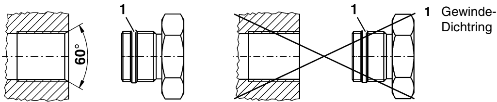
Bild 1: Richtig: Muttergewinde anfasen Bild 2: Falsch
