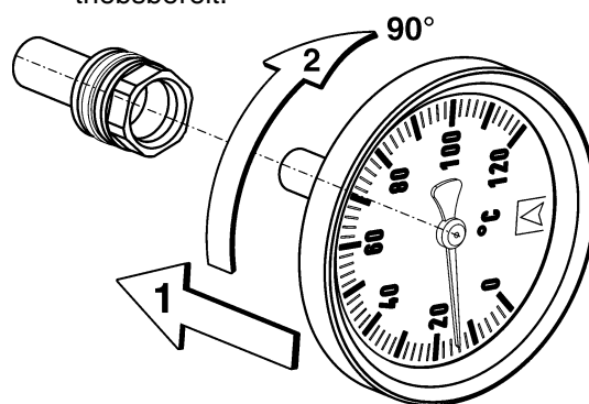
Bild 3: Montage
