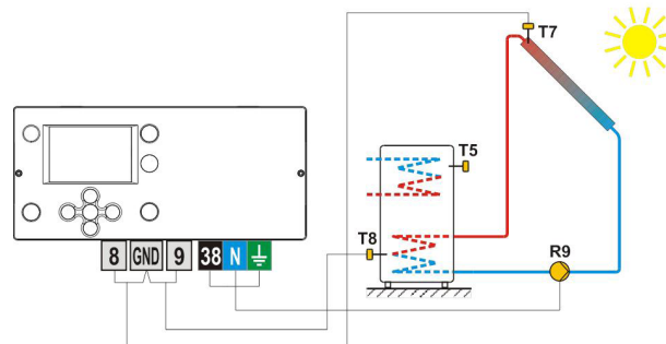
Bild 1- Brauchwassererwärmer
