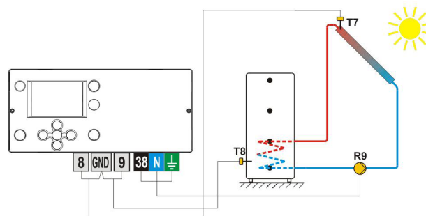
Bild 2- Wärmespeicher
