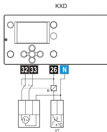
Variante 2: Schließung des Mischventils bei Überschreitung der Temperatur.
