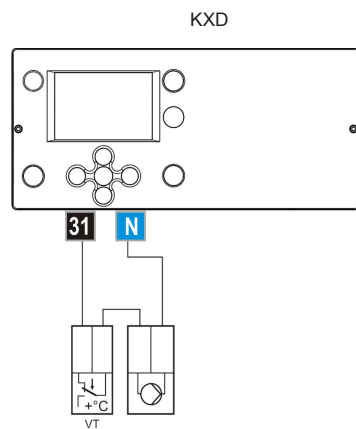
Variante 1: Abschaltung der Umwälzpumpe bei Überschreitung der Temperatur.
