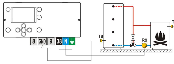
Bild 2- Wärmespeicher
