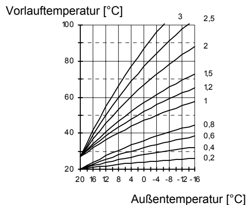
Heizkurvendiagramm (Einstellhilfe)
