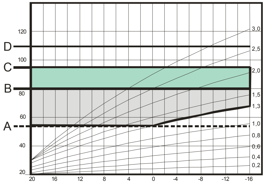
Heizkurvendiagramm (Einstellhilfe) Außentemperatur [°C]
