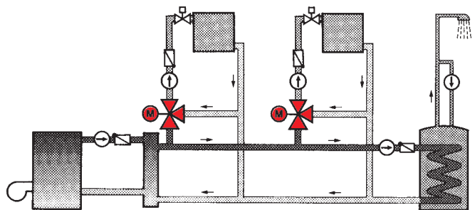
Ein-/Mehrkreisanlagen mit Dreiwegemischer und Hydraulischer Weiche
