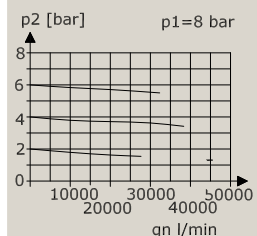
Durchflusscharakteristik
