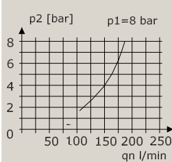
Öler-Ansprechgrenze
