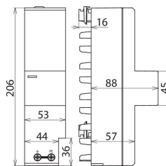
Maßbild DSH ZP TT 255
