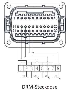
Abb. 6.17 Wechselrichter - RRCR-Verbindung
