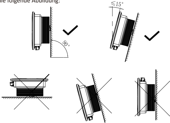
Abb. 5.1 Installationsschema
