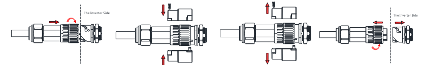
Abb. 6.3 Anschlusschema der AC-Klemme
