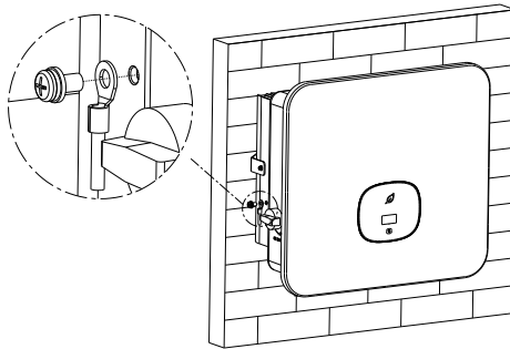
Abb. 6.1 Erdungsschema
