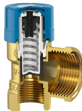
Bild 3: Schnittmodell Membransicherheitsventil 1/2" – 1"
