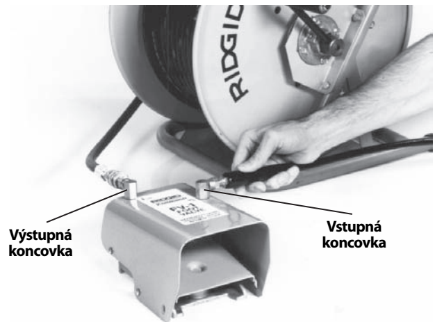
Obrázok č. 11 – Pripojenie nožného ventilu
