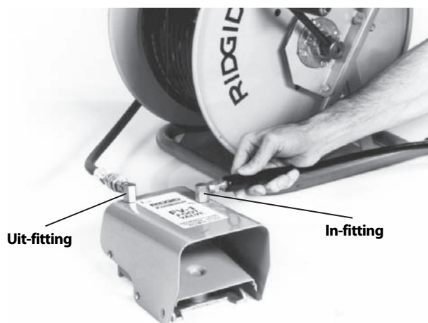
Figuur 11 – Voetklepaansluiting
