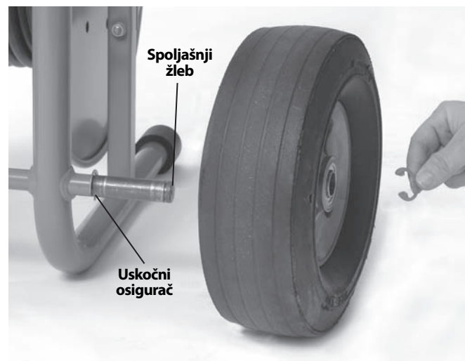
Slika 4 – Sklop KJ-2200
