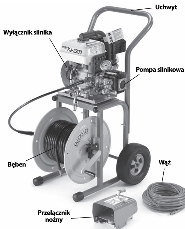
Rysunek 1 - Przepychacz wodny KJ-2200
