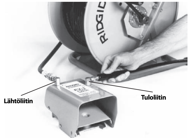
Kuva 11 – Jalkaventtiiliin liittäminen
