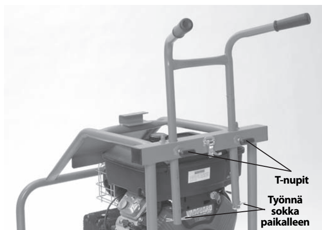
Kuva 5 – KJ-3100 Kahva-asennus
