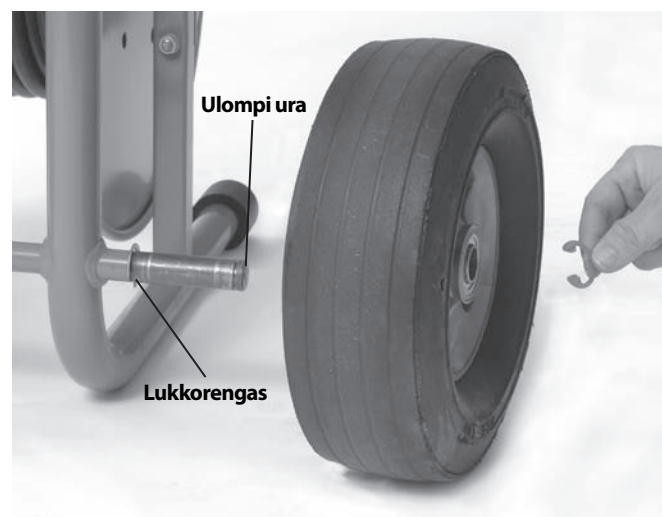
Kuva 4 – KJ-2200:n asennus
