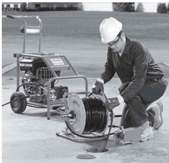
Figur 14 – Passende betjeningsstilling
