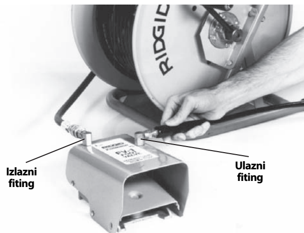
Slika 11 – Priključak nožnog ventila
