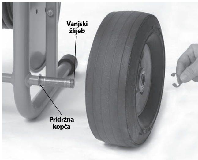
Slika 4 – Sastavljanje modela KJ-2200
