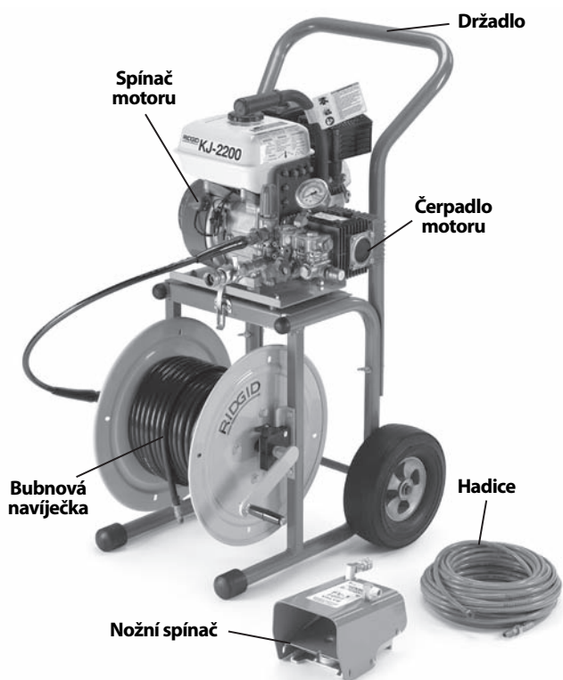
Obrázek 1 – KJ-2200 Tlaková vodní čistička
