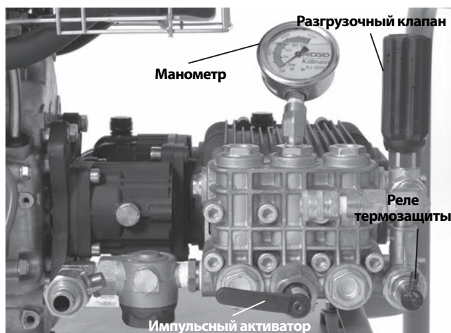
Рис. 13 - Средства управления
