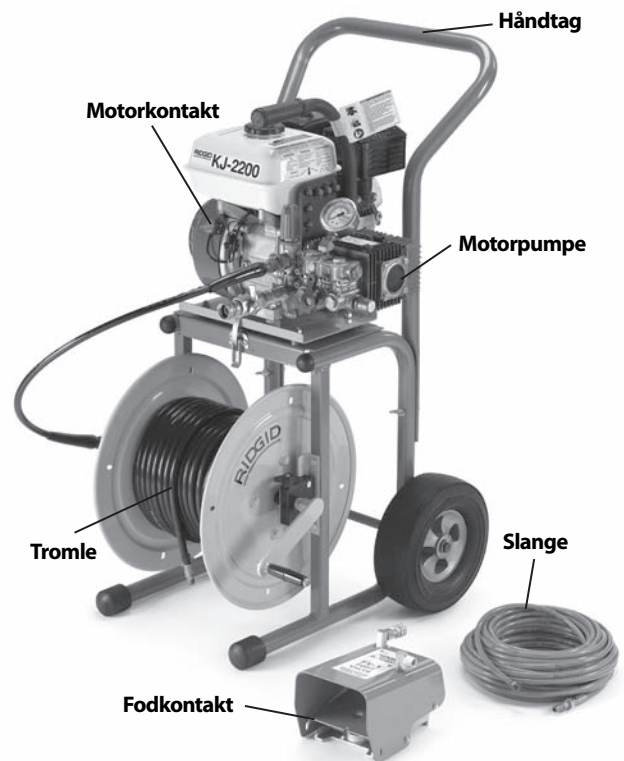
Figur 1 – KJ-2200-højtryksrensere
