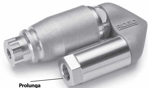
Figure 12 – Iniettore con prolunga RR3000
