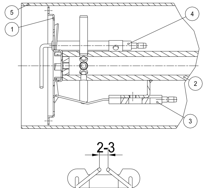
Abb. 17 Zündelektrodenpositionierung
