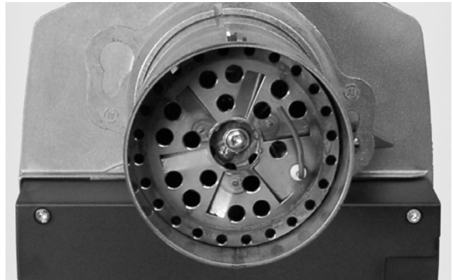
Abb. 19: Position Ionisationselektrode
