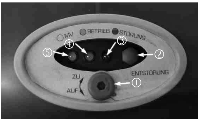
Abb. 5: Lampenfeld SGN(F) 120H
