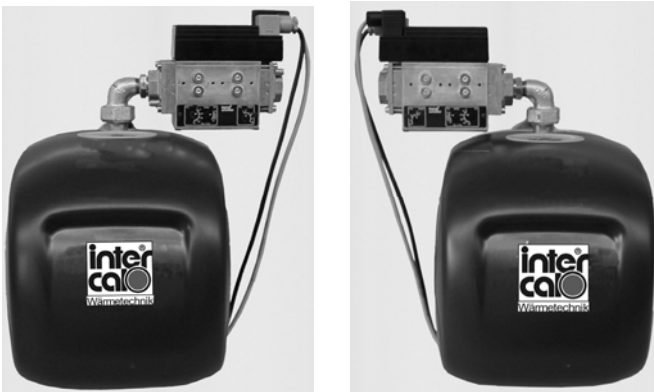
Abb. 3: Montage Gasarmatur
