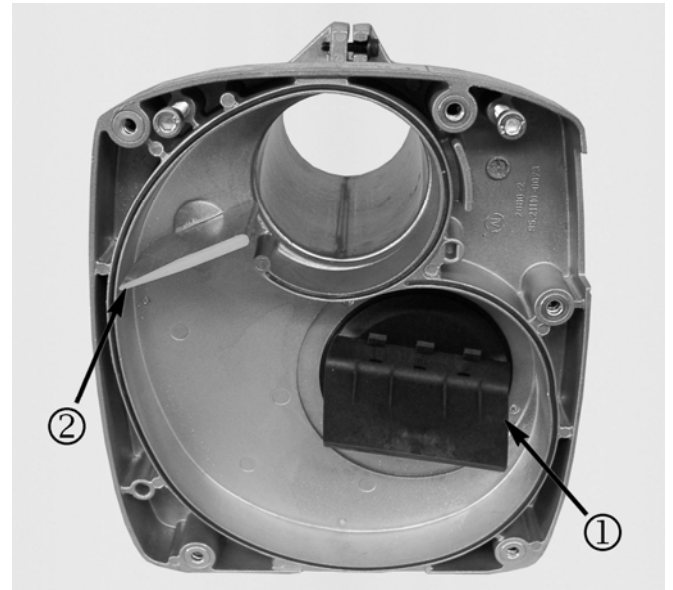
Abb. 6: Lufteinlaufdüse mit Winkel
