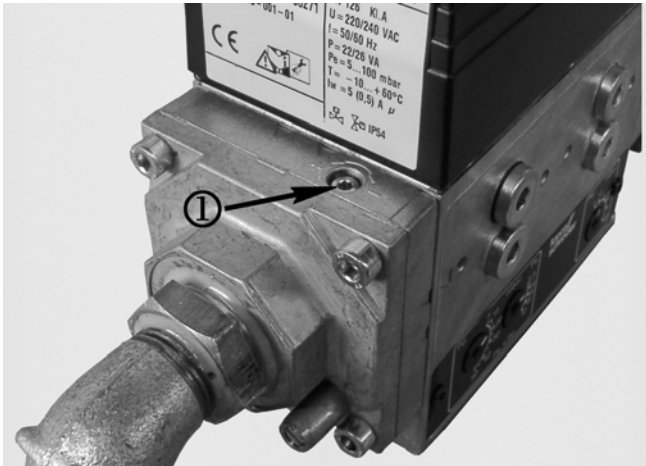
Abb. 14: Einstellschraube ① drehen: Nach rechts (-) = Drossel schließen Nach links (+) = Drossel öffnen
