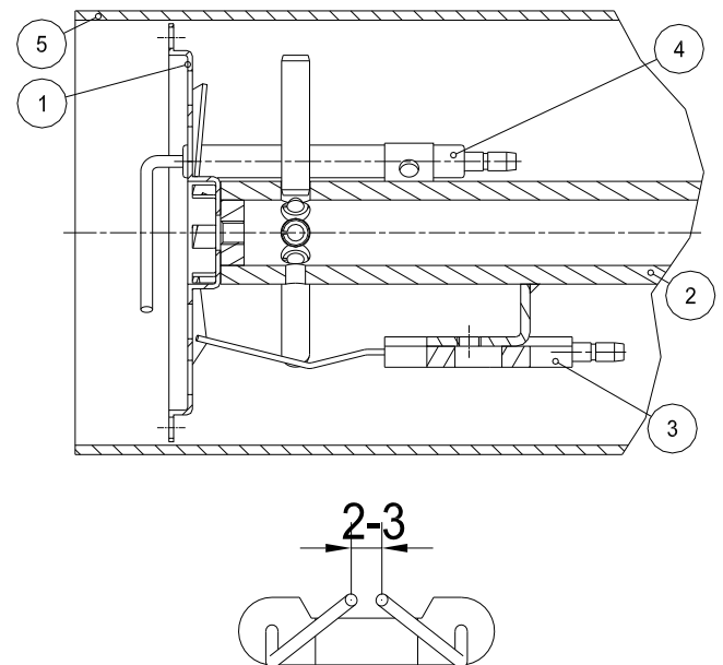
Abb. 17 Zündelektrodenpositionierung
