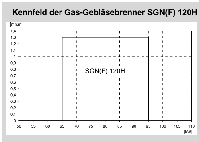
Abb. 28: Legende: mbar = zulässiger Feuerraumdruck kW = Kesselleistung [kW] (Erdgas H)
