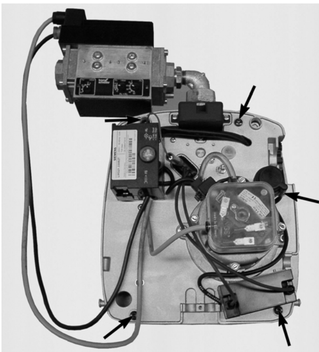
Abb. 15: Gehäusedeckel mit 5 Schnellverschluss-Schrauben
