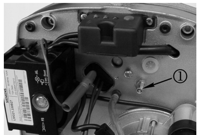
Abb. 7: ① Messanschluss zur Bestimmung der Gebläsepressung
