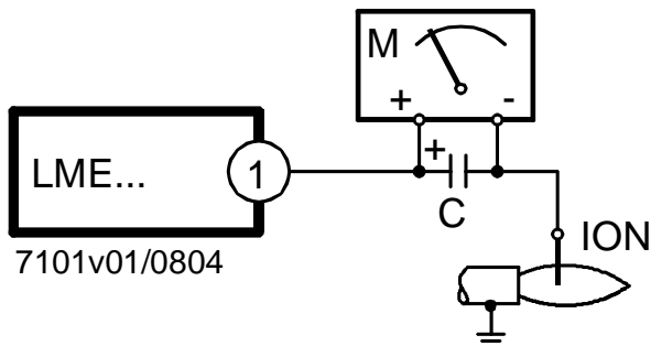
Abb. 18: Legende Mess-Schaltung
