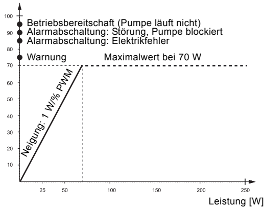
Abb. 8 PWM-Rückmeldesignal - Leistungsaufnahme
