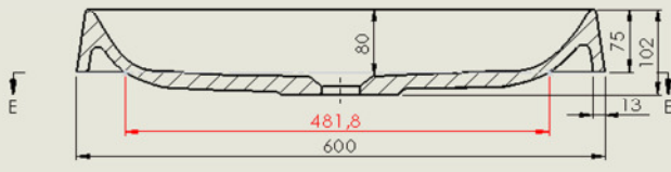
E-E
