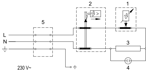
Elektroschaltbild
