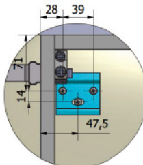
DETTAGLIO A
