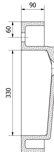
SEZIONE B-B
