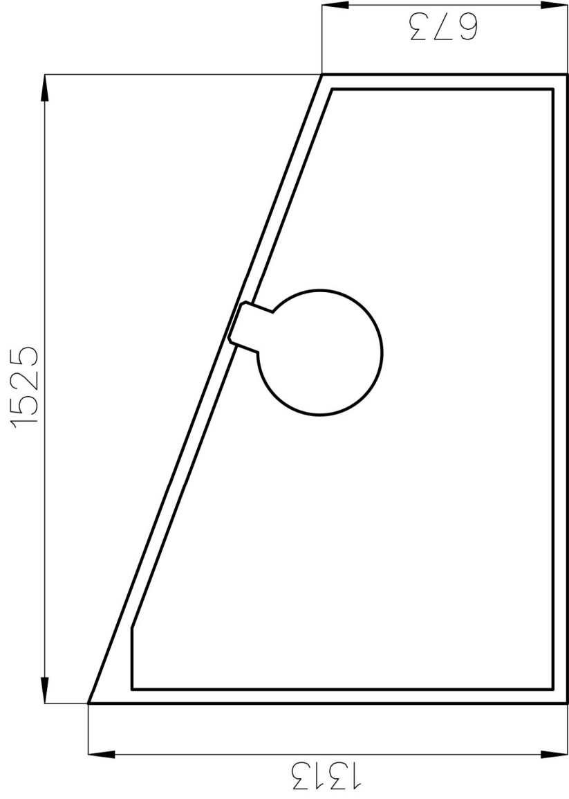
Draufsicht
