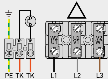
TCBT Modelle 3~ 400 V, 50 Hz, alle außer: TCBT/2-250/H
