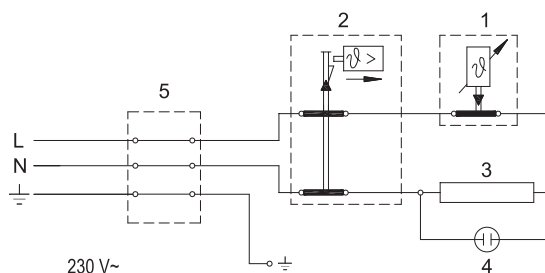
Elektroschaltbild
