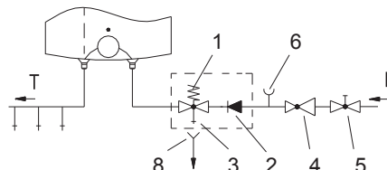
Sous évier
