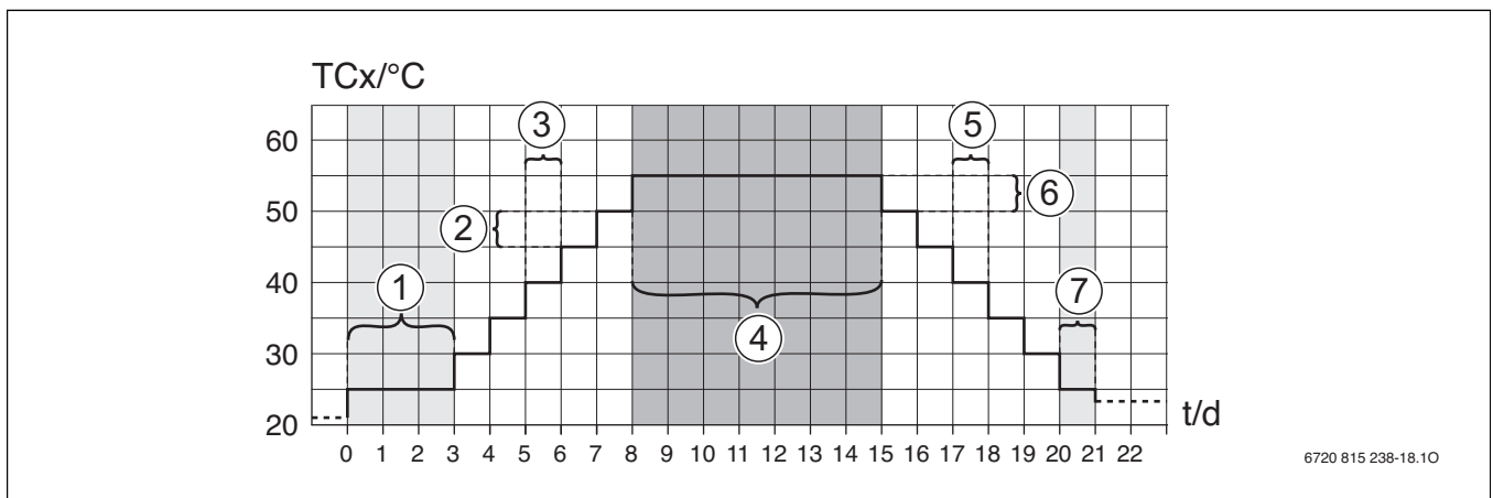
Bild 13 Ablauf der Estrichrocknung mit Grundeinstellungen
