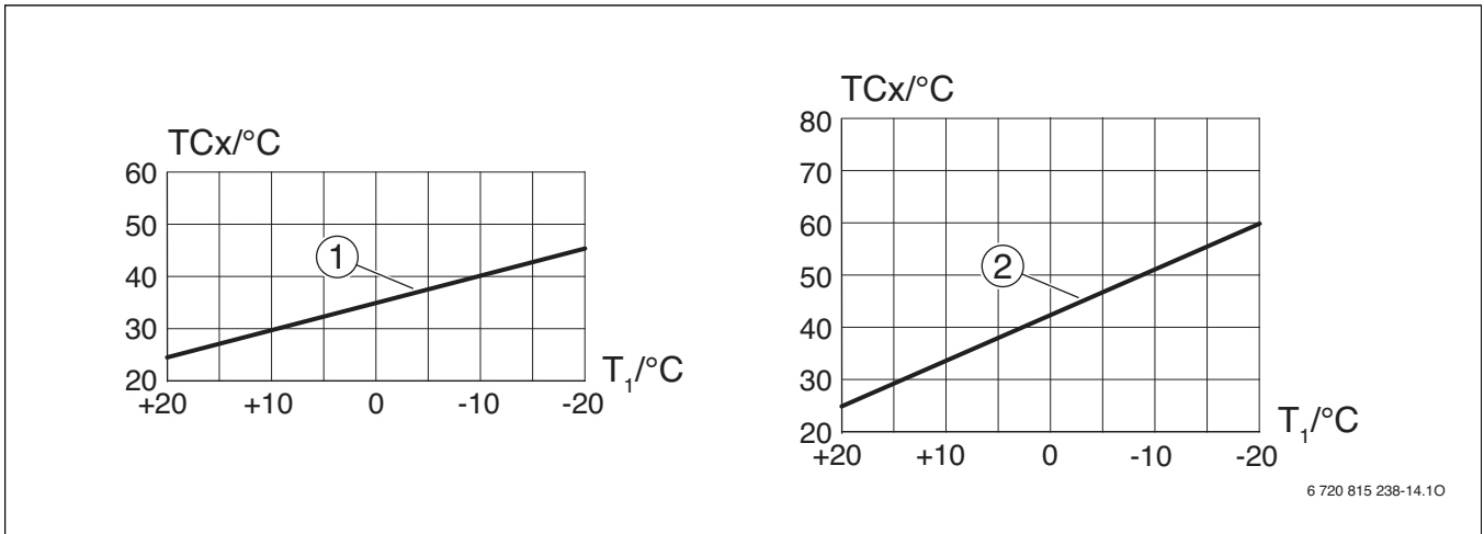
Bild 10 Einstellungen der einfachen Heizkurven
