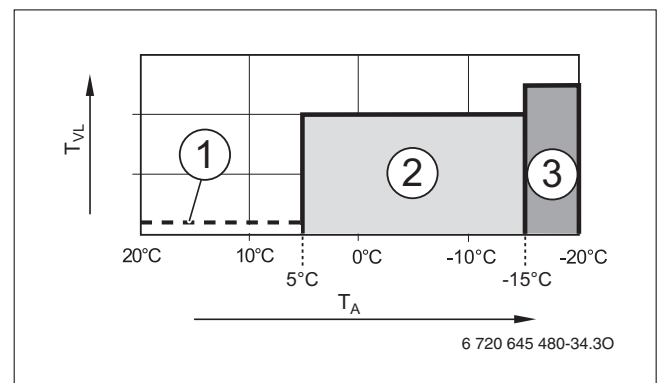
Bild 12 Auswirkung bei Einstellung - 15 °C
