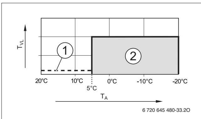
Bild 11 Auswirkung bei Einstellung Aus (Grundeneinstellung)
