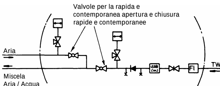
Figura 18: Dispositivo di miscelatura Aria compressa / Acqua
