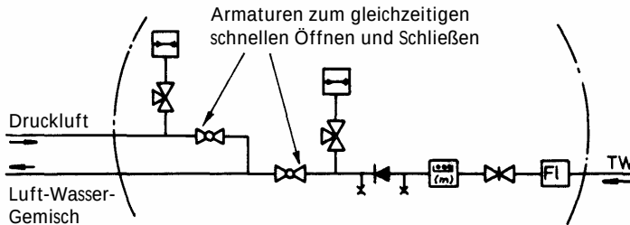
Bild 18: Druckluft-Wasser-Mischvorrichtung
