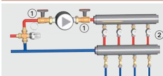
Vorlauftemperaturregelung bei Fußboden-Heizkreisverteiltern mit Thermostat-Kopf K mit Anlegefühler.
