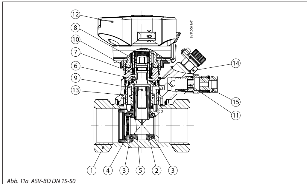
Abb. 11a ASV-BD DN 15-50
