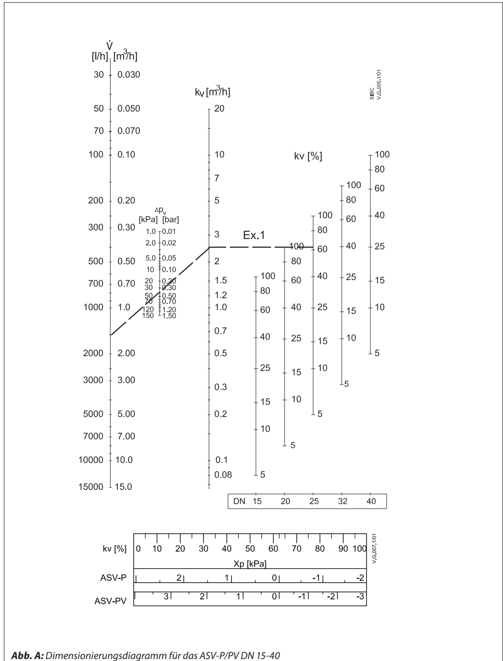
Abb. A: Dimensionierungsdiagramm für das ASV-P/PV DN 15-40
