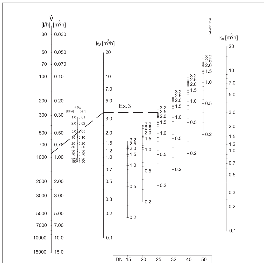
Abb. D: Dimensionierungsdiaagramm für das ASV-I, DN 15-50
