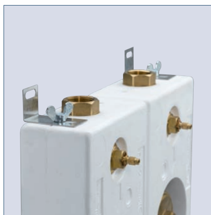
Befestigungsdarstellung inkl. Montagewinkel
