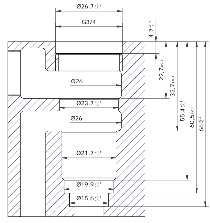
A-A (1.5:1)
