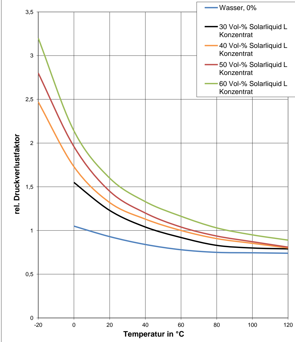
rel. Druckverlustfaktor von Solarliquid L Konzentrat/ Wassermischungen in Abhängigkeit von Temperatur und Konzentration
