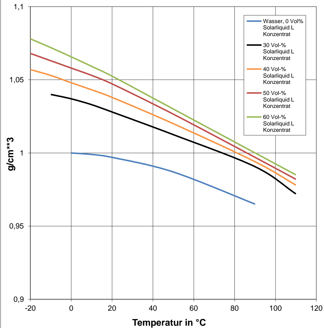
spez. Dichte Solarliquid L Konzentrat/ Wassermischungen in Abhängigkeit von Temperatur und Konzentration
