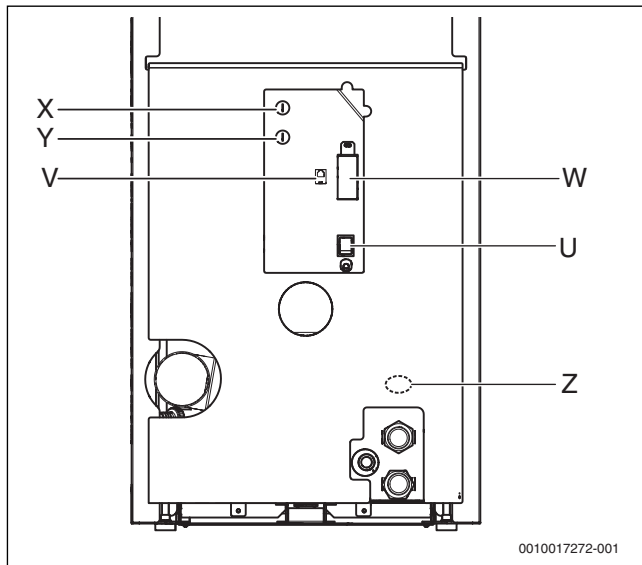
Bild 16 Anschlüsse Rückseite
