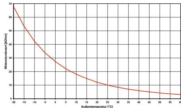
Abb. 8.1: Fühlerkennlinie NTC-10
