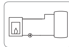
System 5: Kaminofen (ohne Mischer-Darstellung)
