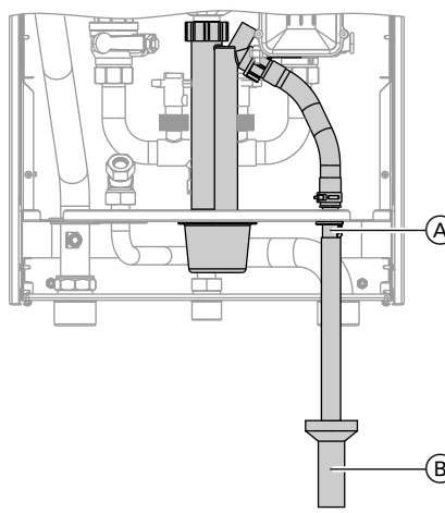
Vitodens 200-W, 69, 80 und 99 kW
