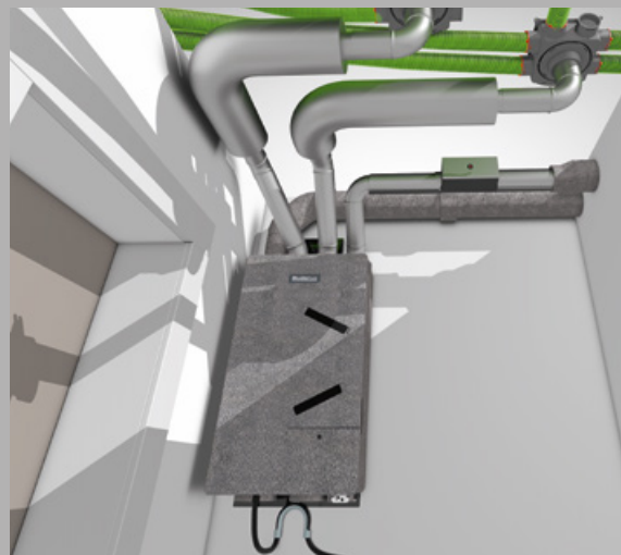
Einbausituation Wand
